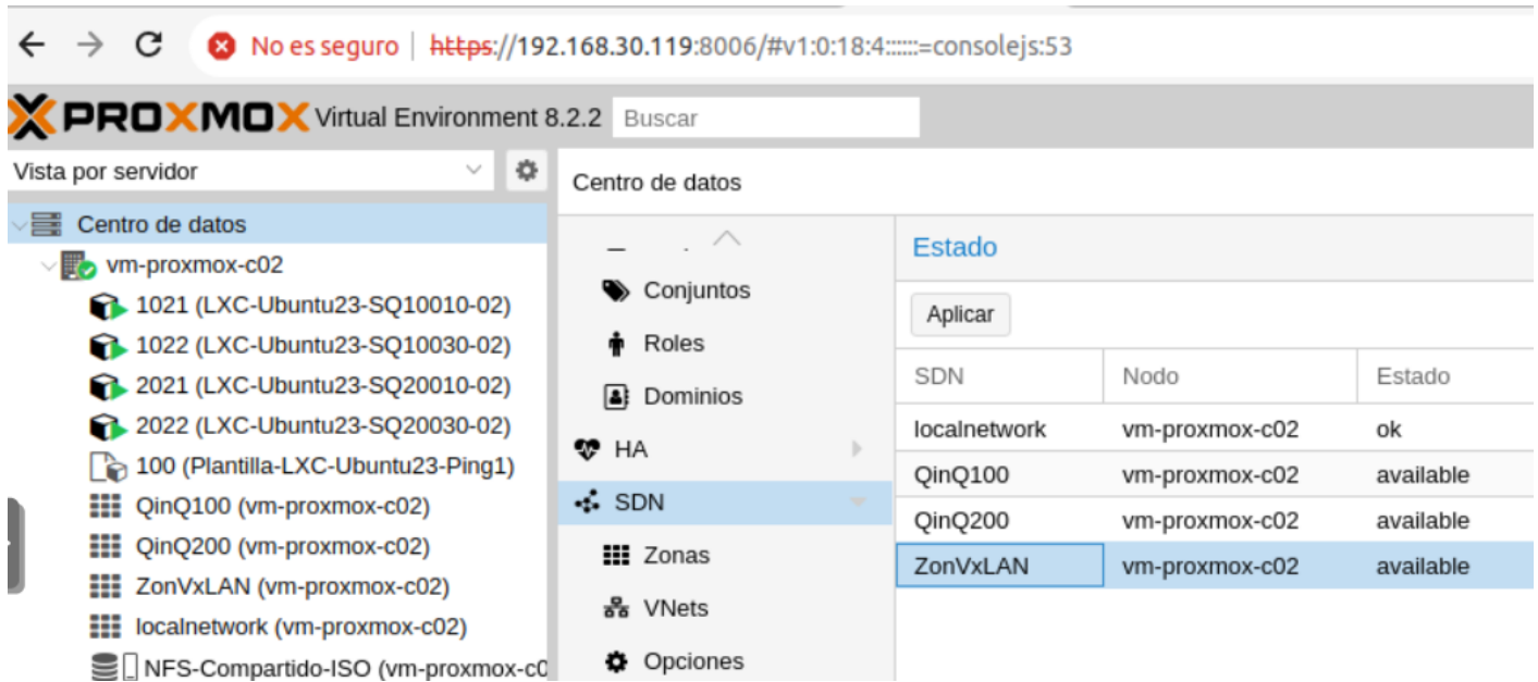
Imagen de elaboración propia: Creación de Zona SDN del tipo VxLAN en el nodo c02 de Proxmox ( CC BY-NC-SA )
