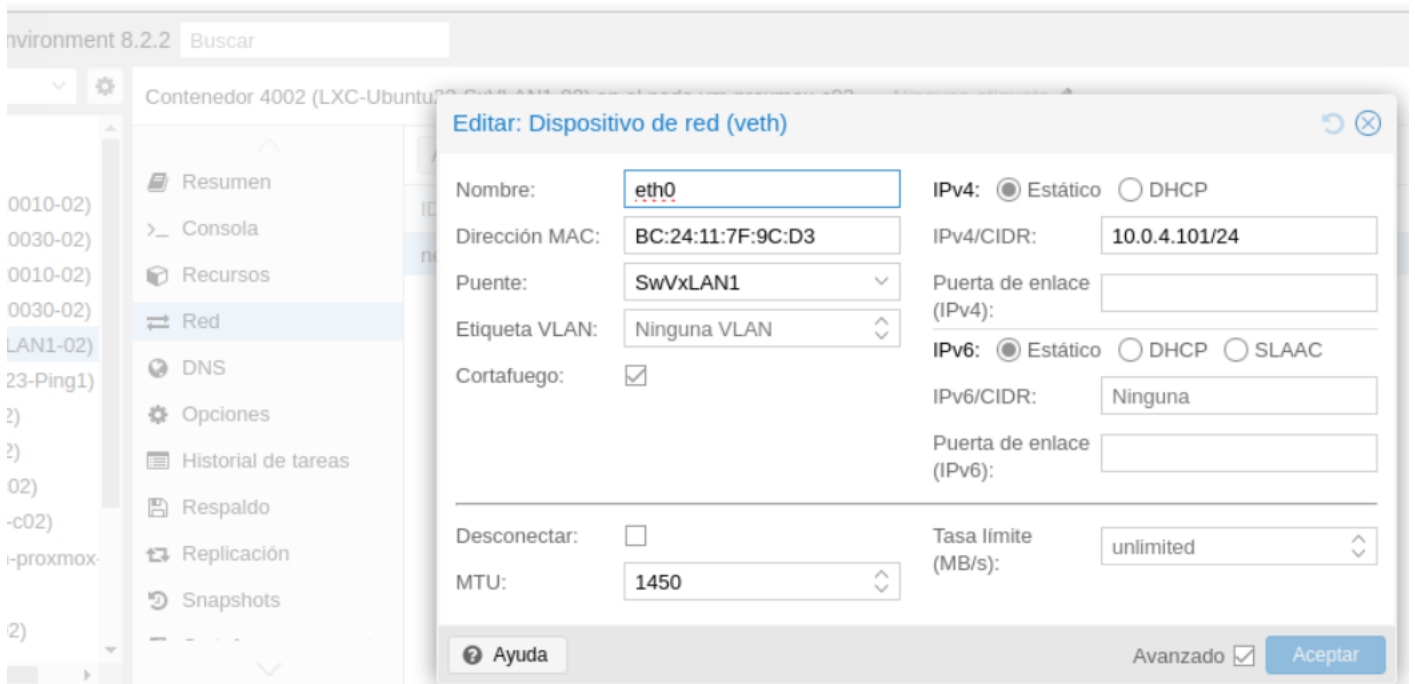
Imagen de elaboración propia: Configuración de red de un contenedor en la VxLAN en el nodo c01 de Proxmox ( CC BY-NC-SA )
