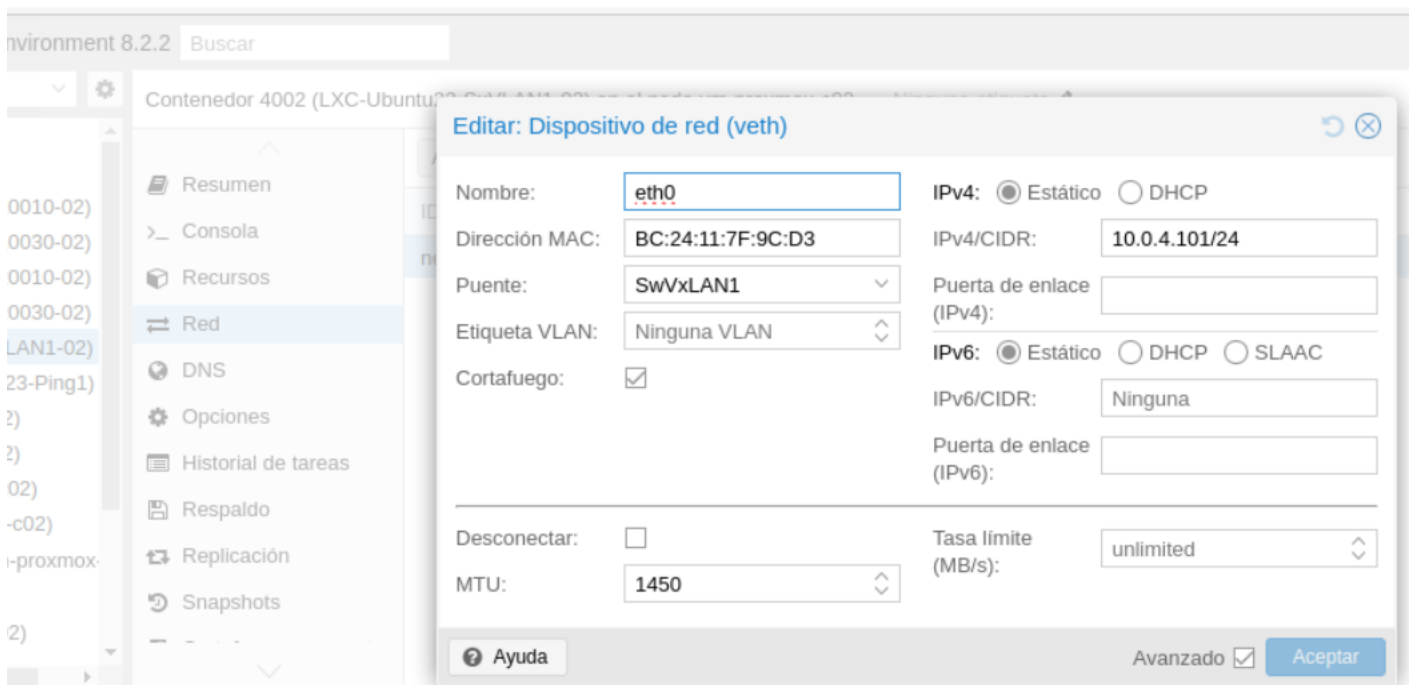
Imagen de elaboración propia: Configuración de red del CT 4002 en el nodo c02 de Proxmox ( CC BY-NC-SA )
