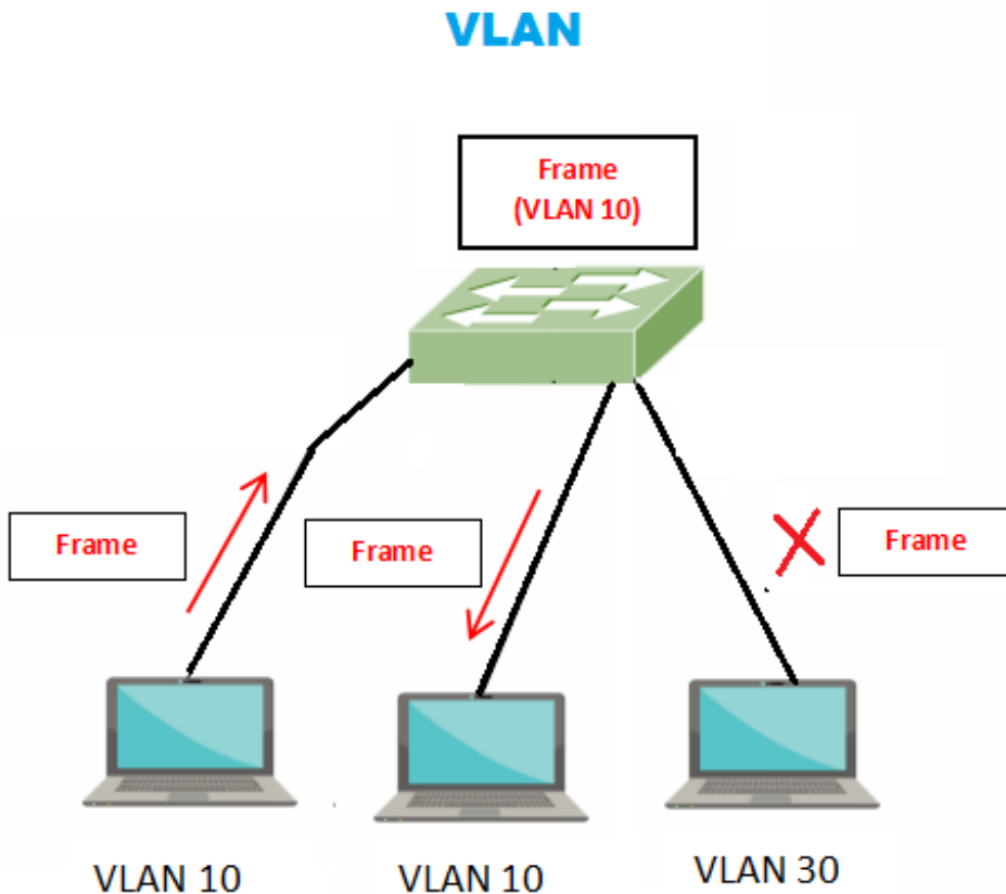
Imagen de elaboración propia · Esquema de una VLAN ( CC BY-NC-SA )
