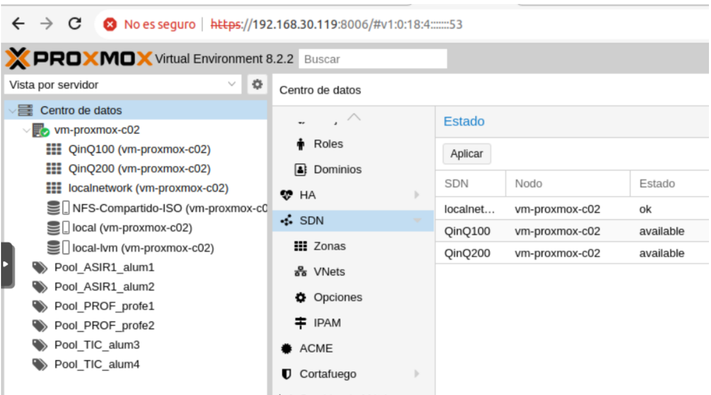
Imagen de elaboración propia: Creación de las dos QinQ en el nodo 2 de Proxmox al igual que hemos hecho en el nodo 1 ( CC BY-NC-SA )
