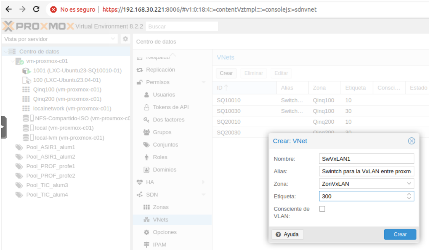
Imagen de elaboración propia: Creación de VNet "SwVxLAN1" ( CC BY-NC-SA )
