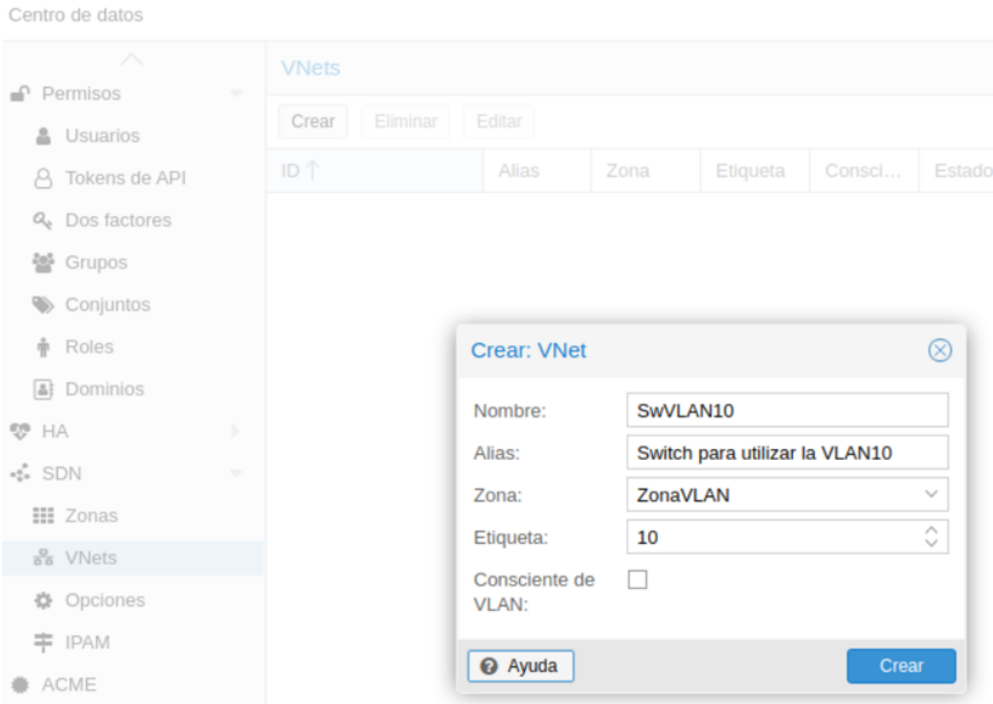
Imagen de elaboración propia: Creación de la VNet "SwVLAN10" ( CC BY-NC-SA )
