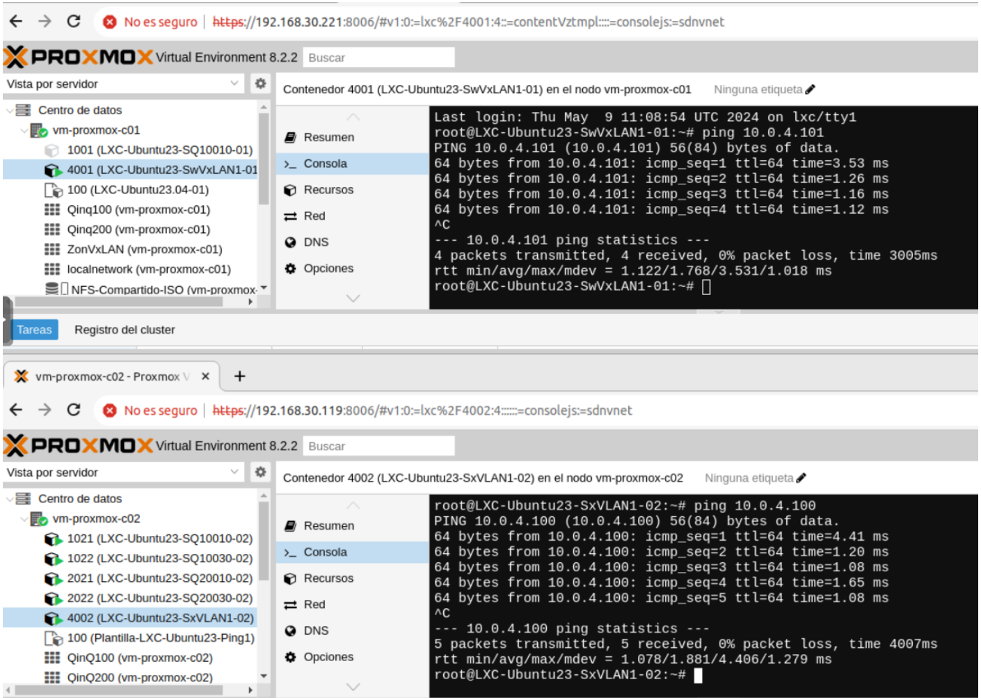
Imagen de elaboración propia: Ping entre CT4001 y CT4002 que se encuentran en dos nodos Proxmox distintos ( CC BY-NC-SA )
